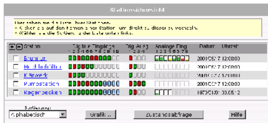
Bild 4.2 Überblick über alle Liegenschaften wie Brunnen, Behälter, Becken und Pumpen.
